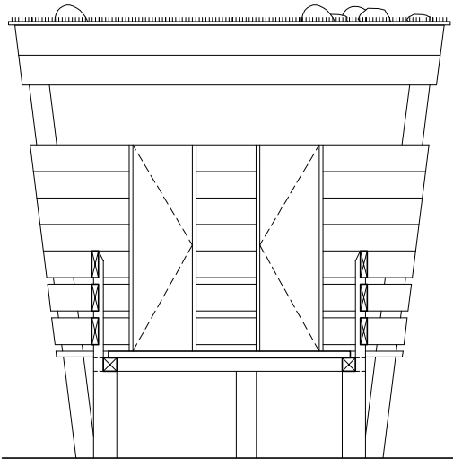
Elevacion frontal Camarines dobles tipo A
