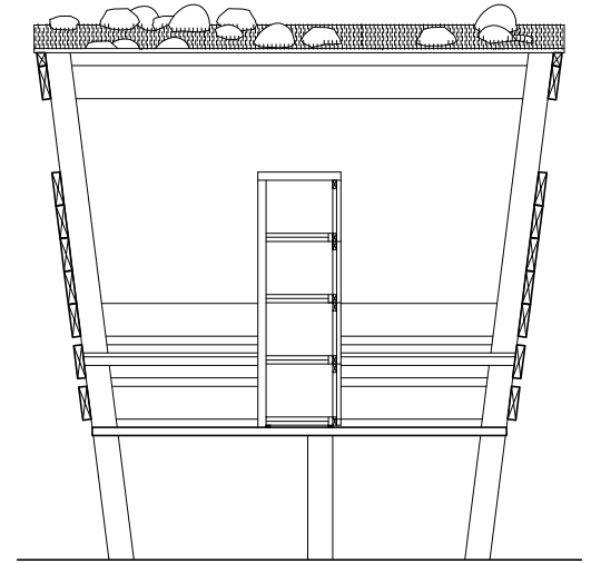
Corte B-B Camarines dobles tipo A
