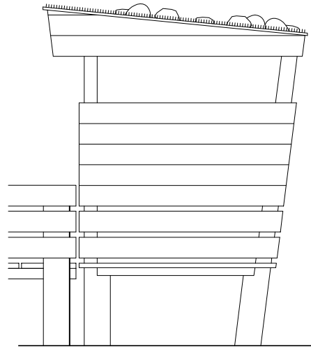
Elevacion lateral Camarines dobles tipo A
