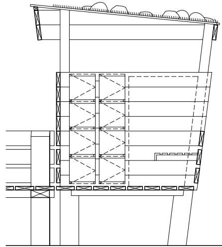
Corte A-A Camarines dobles tipo A
