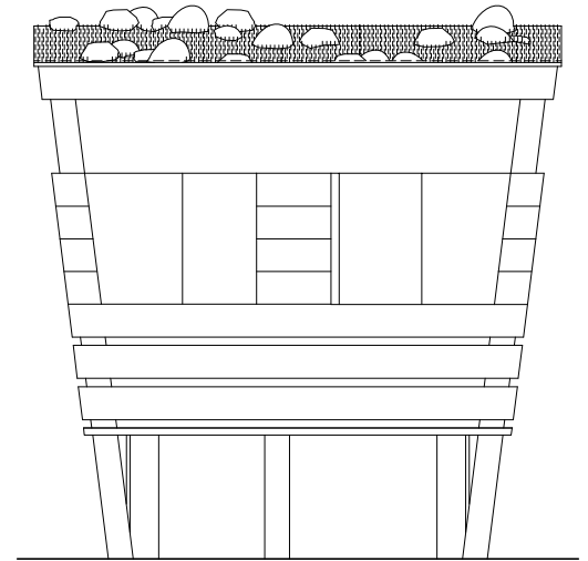
Elevacion posterior Camarines dobles tipo A
