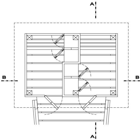
Planta Camarines dobles tipo A
