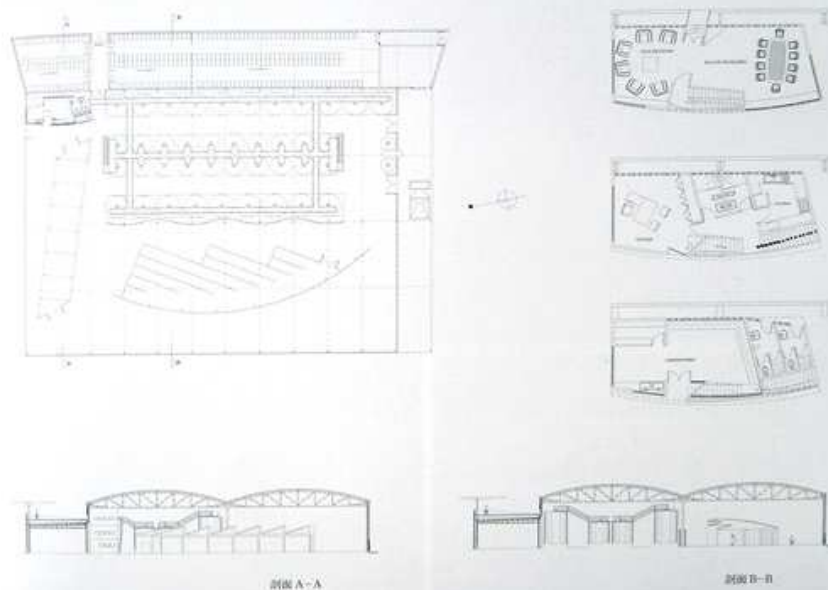
剖面 A-A
