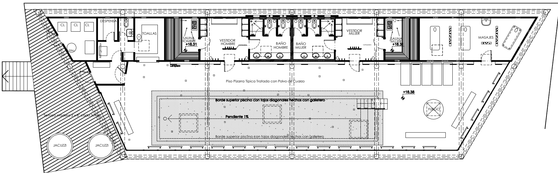
Planta PISCINA
