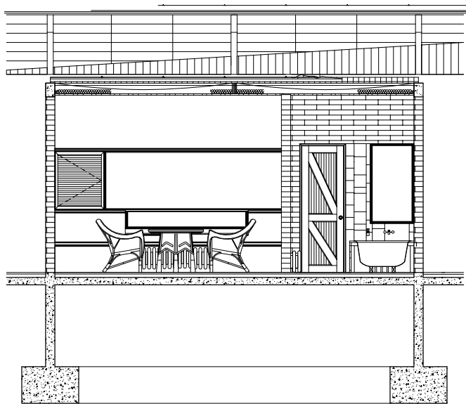
CORTE B-B'
