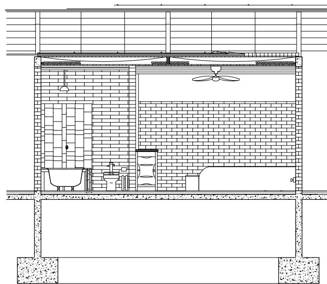
CORTE C-C'
