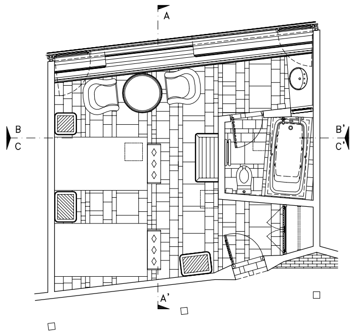
PLANTA
