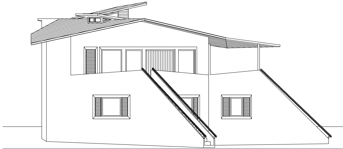
ELEVACION ESTE
