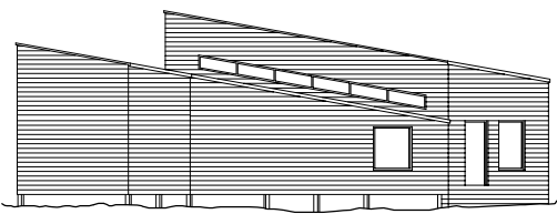
ELEVACION ORIENTE
