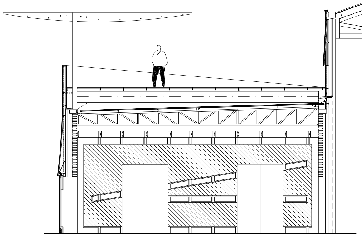
CORTE A-A'
