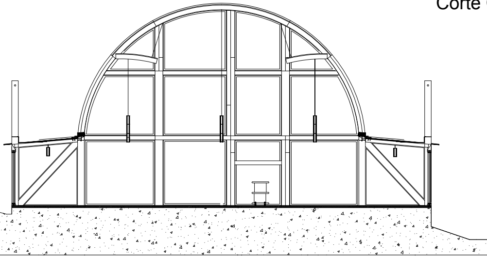
Corte C-C
