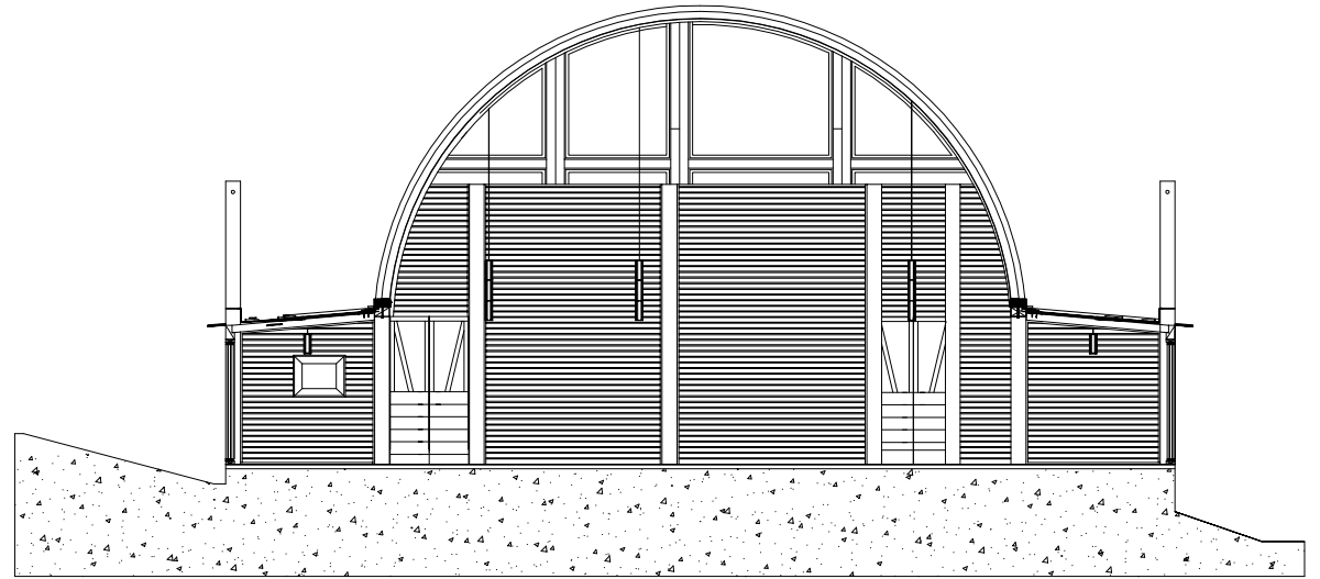
Corte C-C
